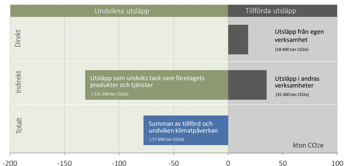
Figur 2. Luleå Energis sammanlagda klimatpåverkan under 2020 uppdelat i direkt klimatpåverkan från Luleå Energis egen verksamhet och indirekt klimatpåverkan som uppstår utanför Luleå Energi. Summan av all klimatpåverkan är negativ vilket innebär att det uppstår mindre utsläpp med Luleå Energis verksamhet än utan.
