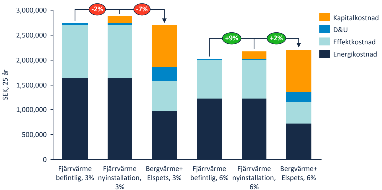
Figur 3 – Livscykelkostnader för alternativa uppvärmningssätt i typiskt flerbostadshus i Vänersborg
