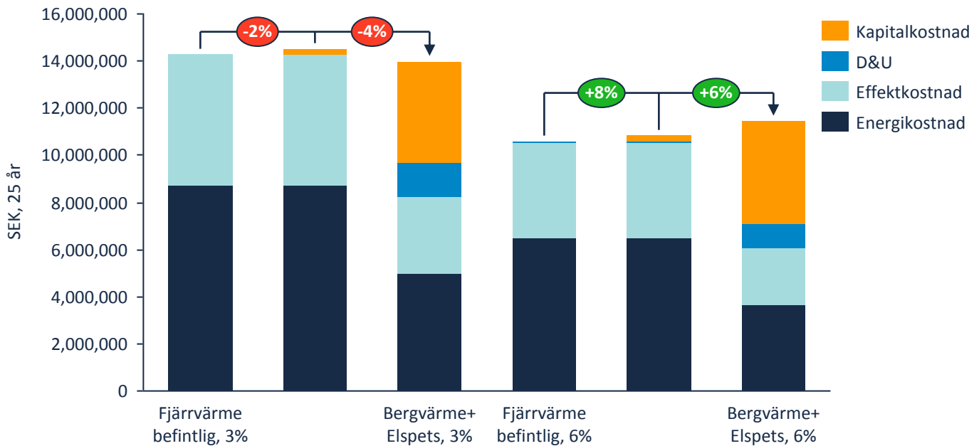
Figur 4 – Livscykelkostnader för alternativa uppvärmningssätt i typisk lokal i Vänersborg.
