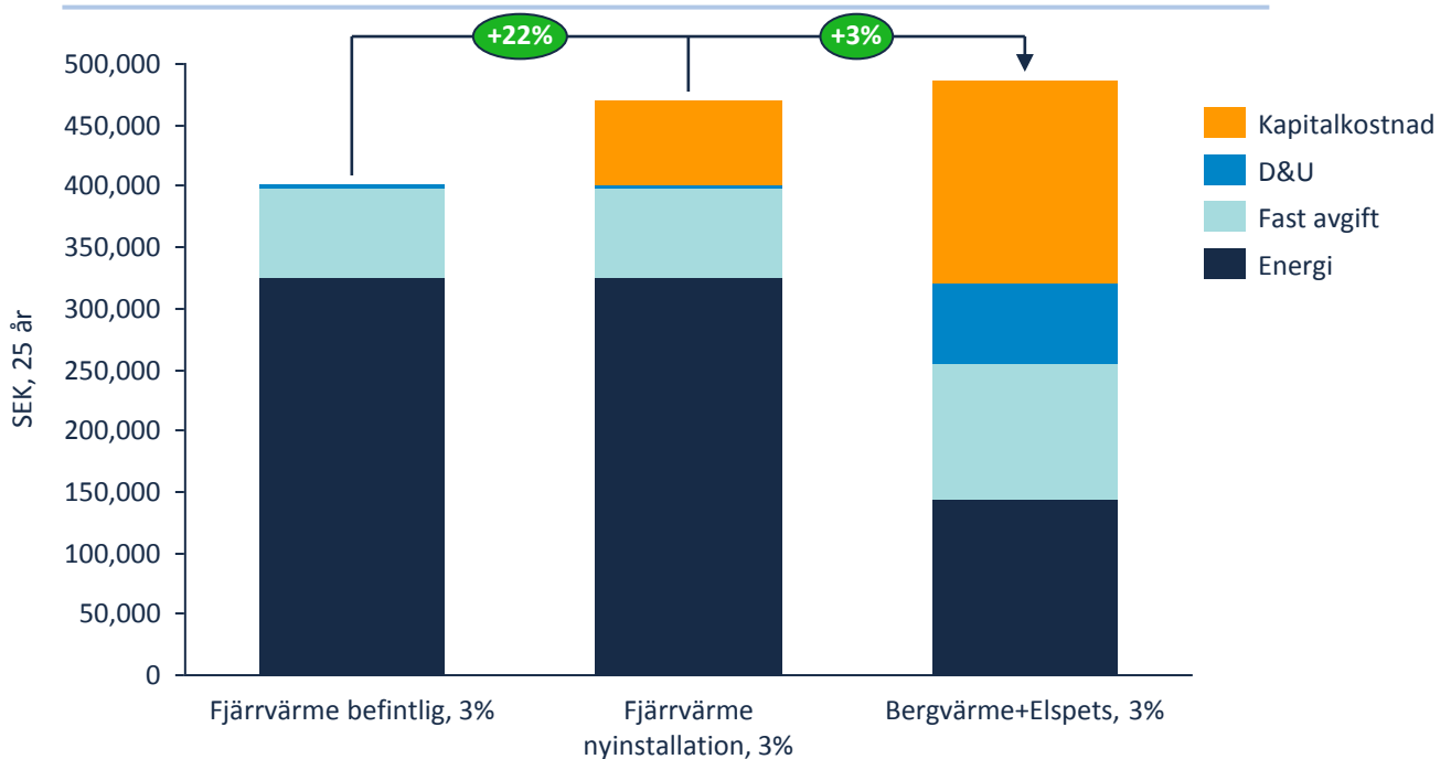
Figur 5 – Livscykelkostnader för alternativa uppvärmningssätt i typiskt småhus Vänersborg
